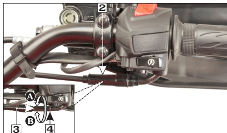
(2) Bota (3) Ajustador (4) Contratuerca (A) Reduce juego libre (B) Aumenta juego libre
