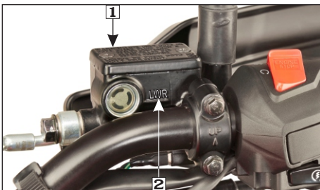
(1) Cilindro principal (2) Marca inferior
