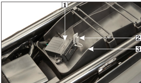
(1) Cargador USB (2) Tapa (3) compartimento del dispositivo USB
