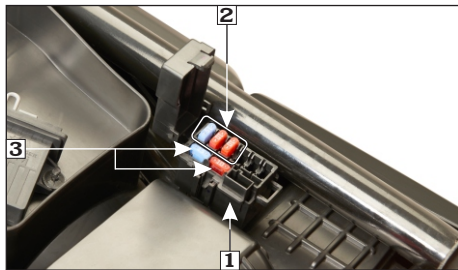
(1) Caja de fusibles (2) Fusible principal (15A, 10A, 10A) (3) Fusible de repuesto (15A, 10A)
