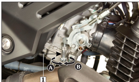
(1) Tornillo de parada del acelerador (A) Aumenta rpm (B) Reduce rpm
