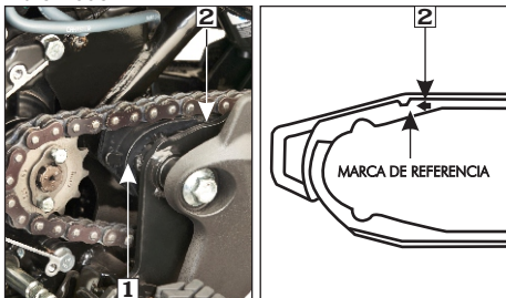
(1) Deslizador de cadena (2) Límite de desgaste
