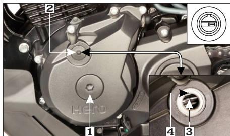
(1) Tapa del orificio del cigüeñal (2) Tapa del orificio de sincronización (3) Marca 'T' (4) Marca de índice
