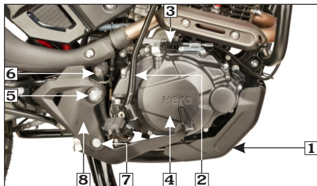
(1) Placa de protección (2) Pedal de arranque (3) Cable del embrague (4) Tapa del cárter derecho (5) Tuerca brazo oscilante (6) Perno de montaje del silenciador (7) Perno de la cubierta del soporte del posapiés del conductor (8) Conjunto de soporte del posapiés
