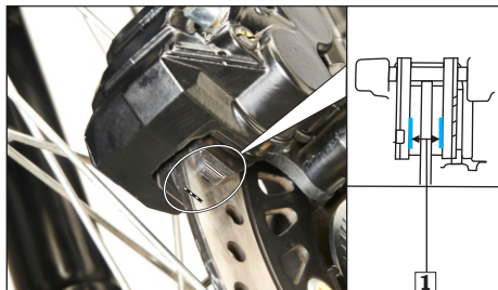
(1) Ranuras indicadoras de desgaste
