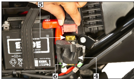
(4) Interruptor magnético de arranque (5) Fusible principal (20A) (6) Fusible de repuesto (20A)
