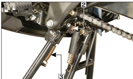
(2) Interruptor soporte lateral (3) Resorte soporte lateral
