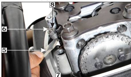
(5) Calibrador de cinta (6) Tornillo de ajuste (7) Vástago de la válvula (8) Tuerca de bloqueo
